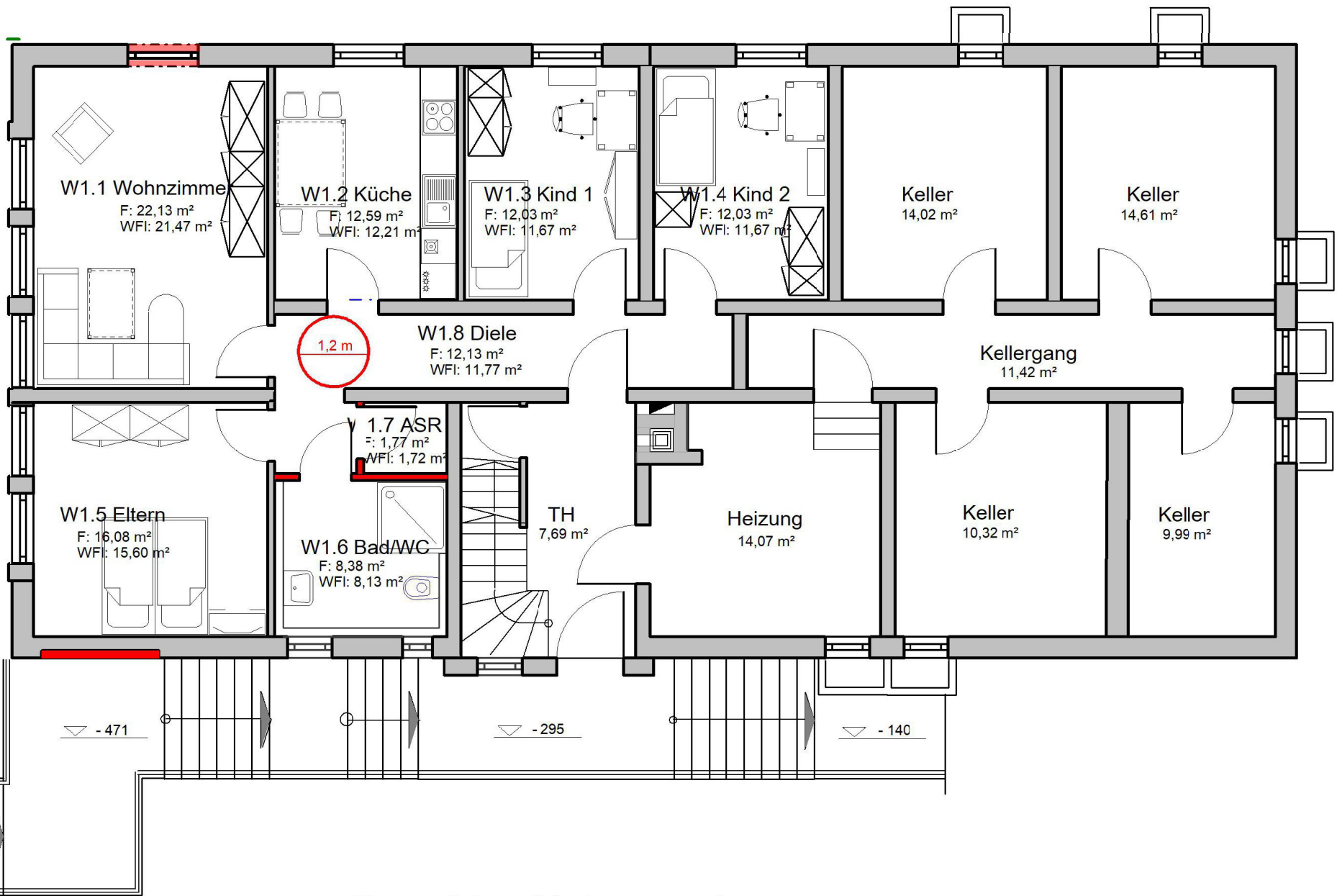
Grundriss Untergeschoss
